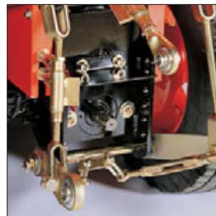
Starke Heckzapfwelle mit Normprofil (zwei Drehzahlen wählbar). Sehr robuste Hinterachse in Blockbauweise. Zuschaltbare Differentialsperre.
